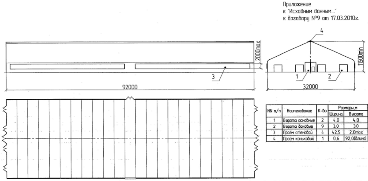
Габаритно-компоновочная схема здания коровника
