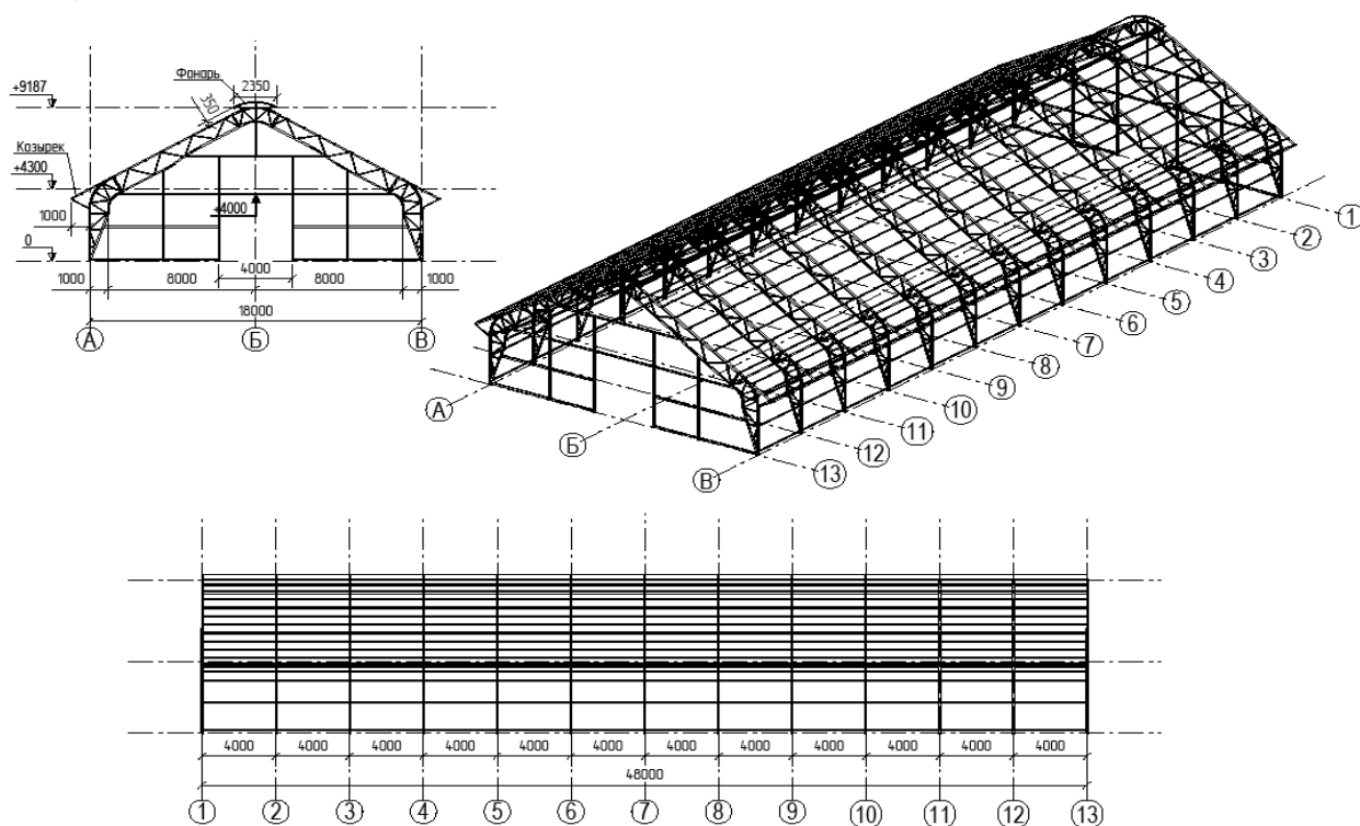
Схема каркаса телятника 18х48х4,3м.
