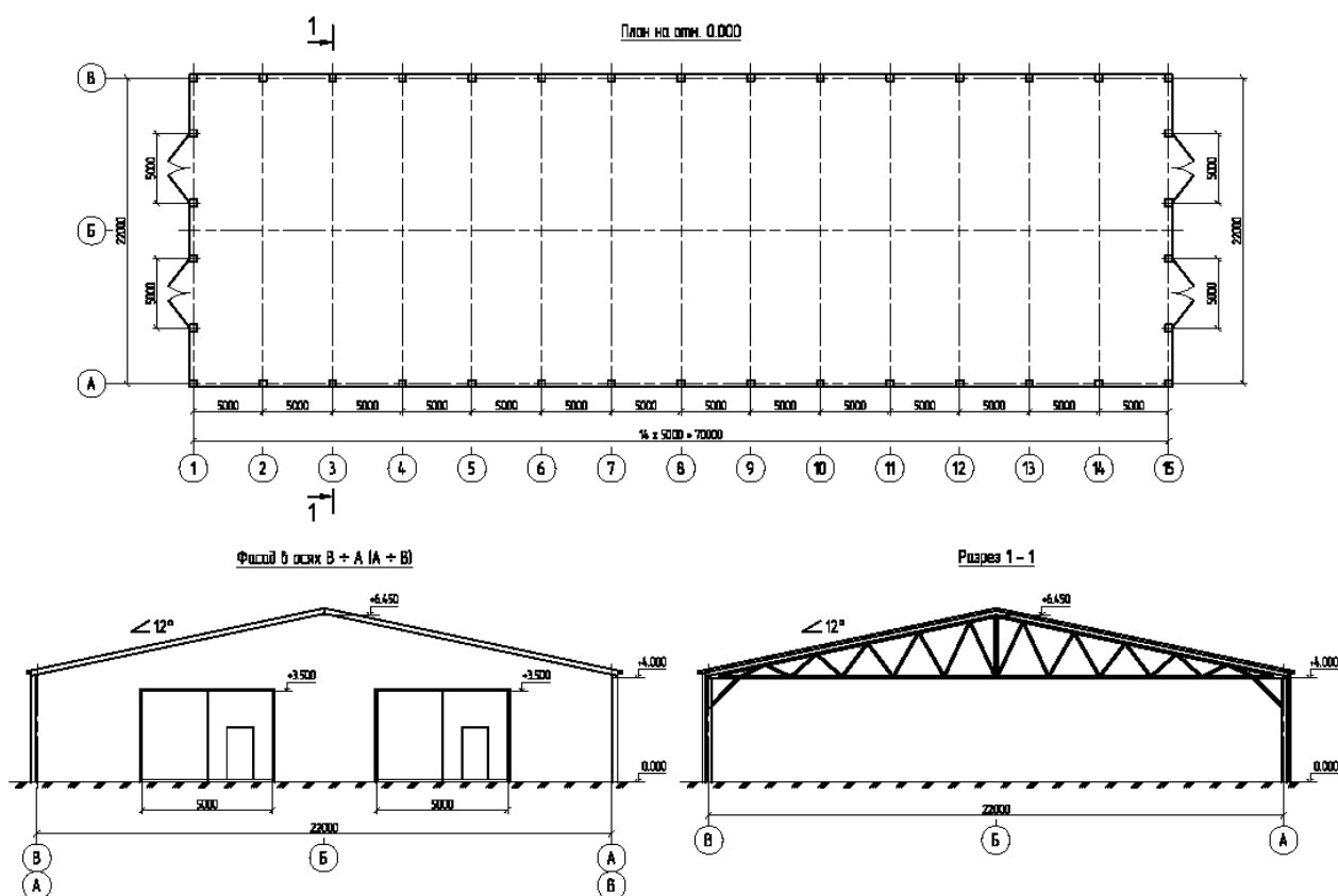
Схема коровника 22.0 х 70.0 х 4.0 м
