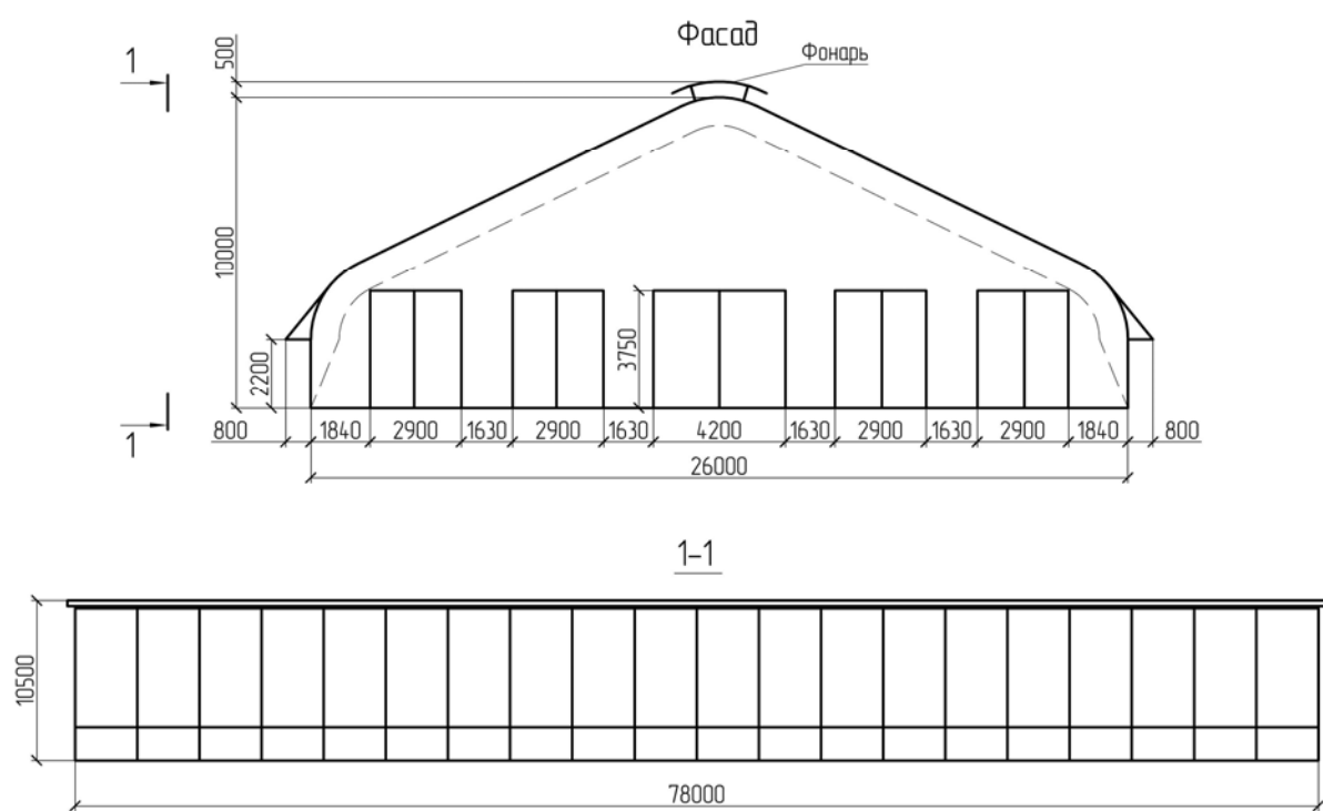
Схема тентового укрытия КРС 26,0х78,0м
